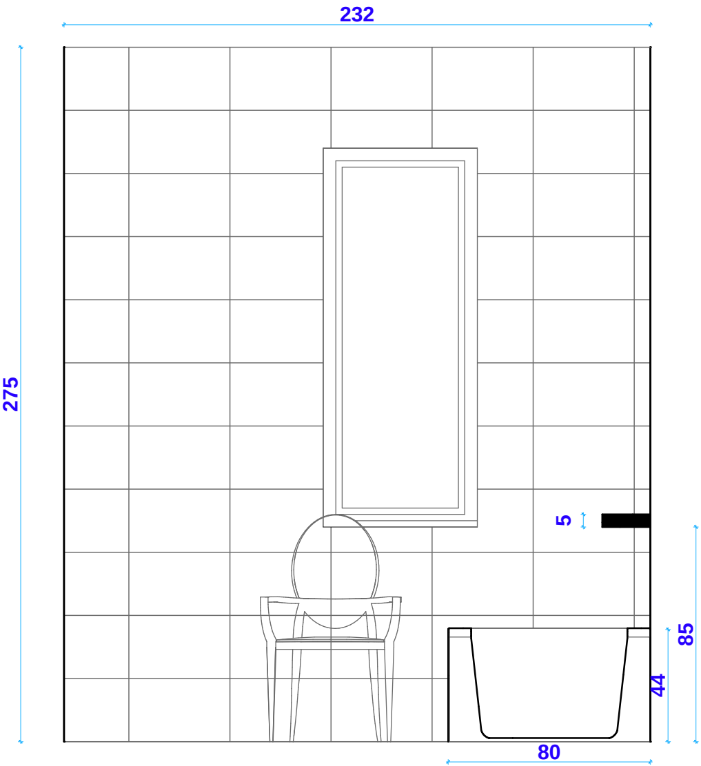
Ściana B
