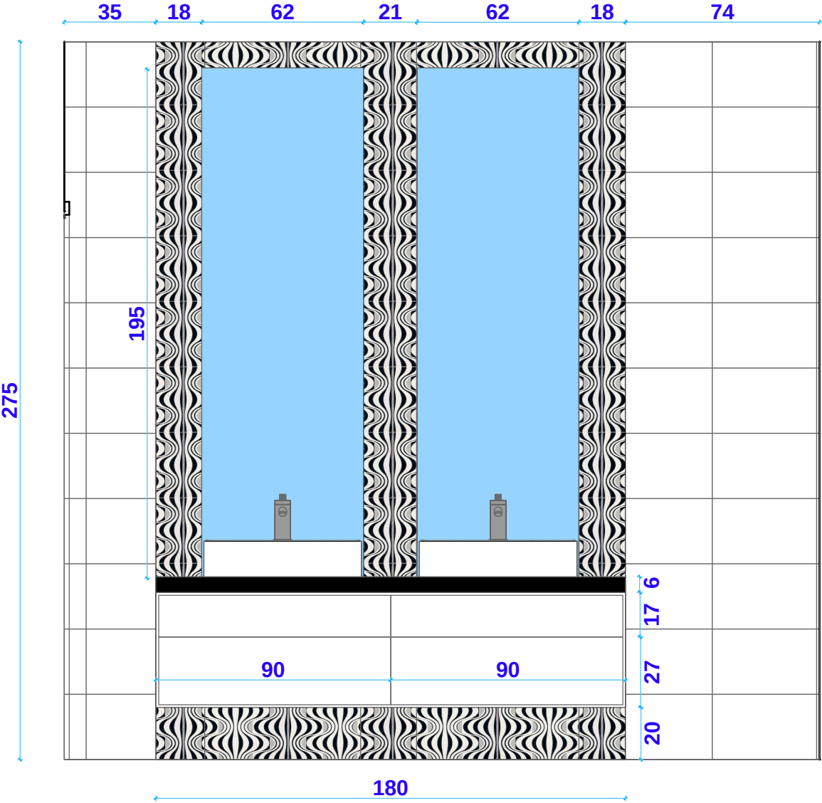
Ściana A
