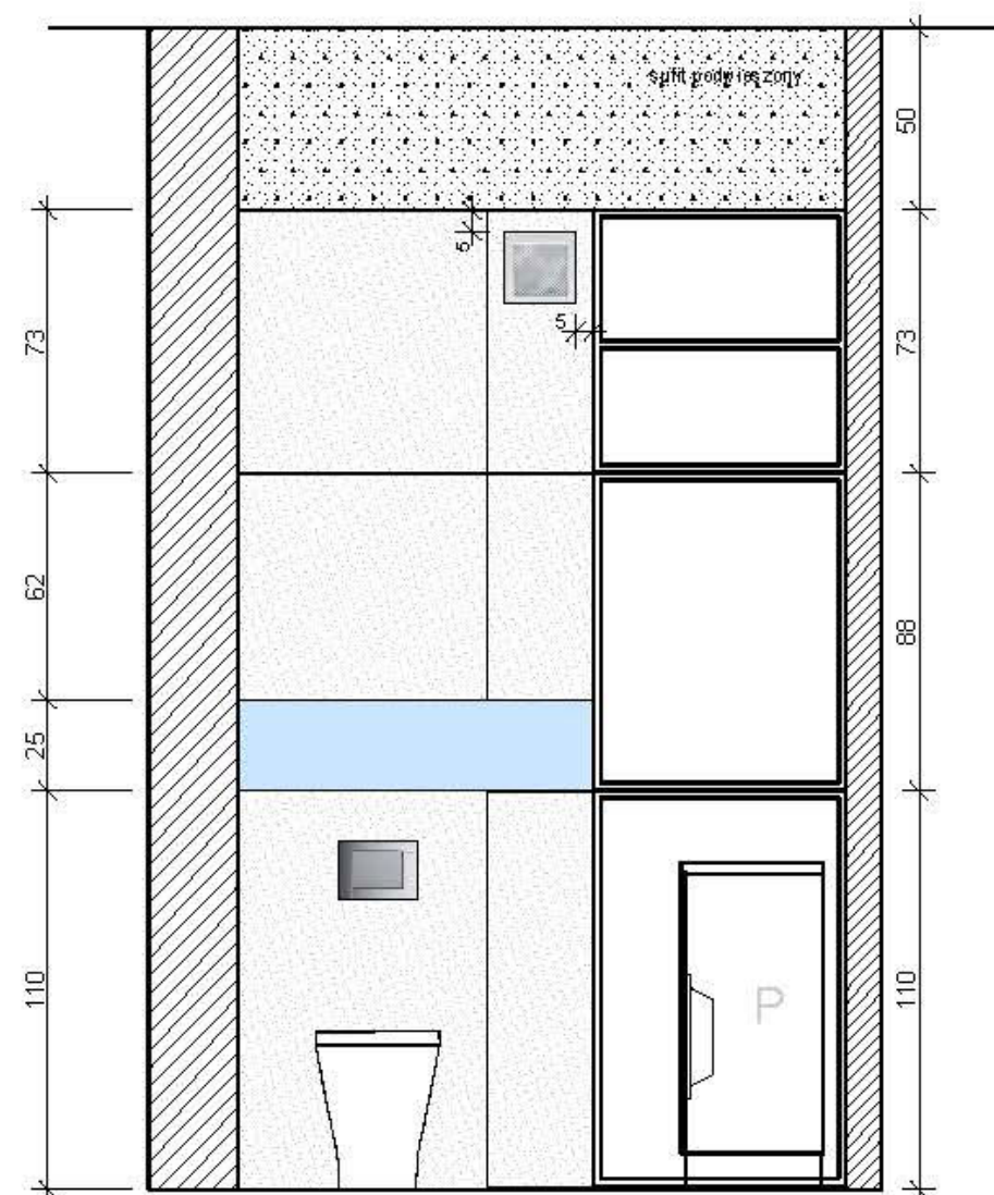
Łazienka 1 - przekrój B1
