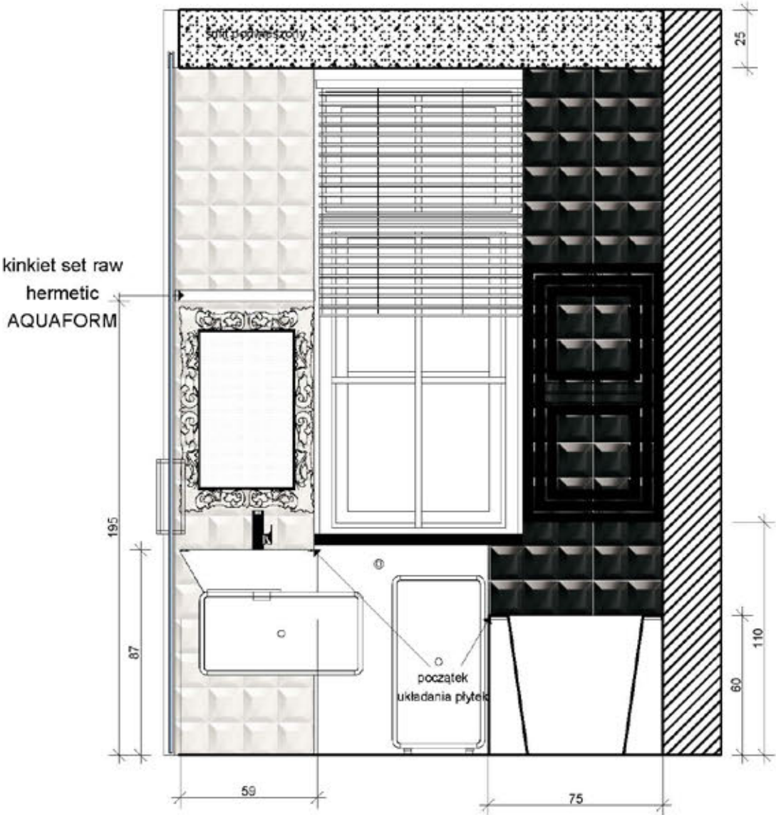
Łazienka 2 - przekrój C1
