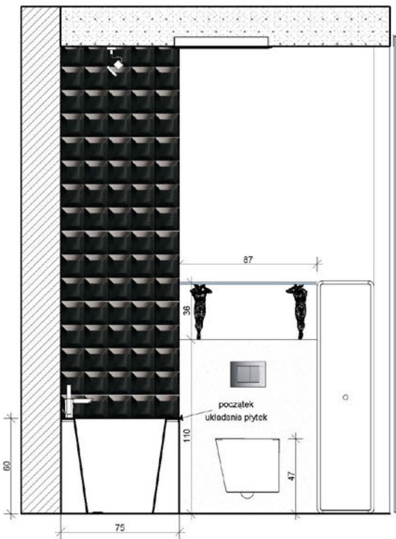
Łazienka 2 - przekrój C3
