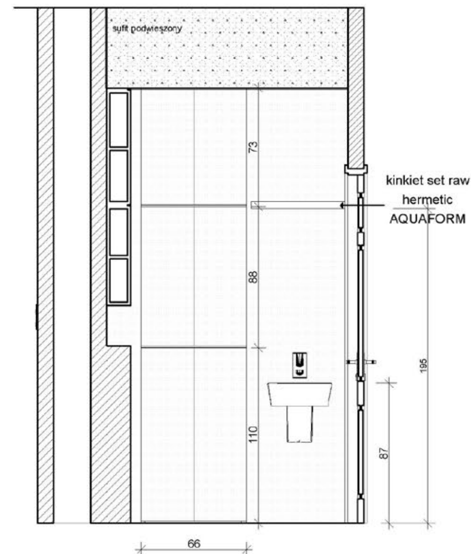
Łazienka 1 - przekrój B2
