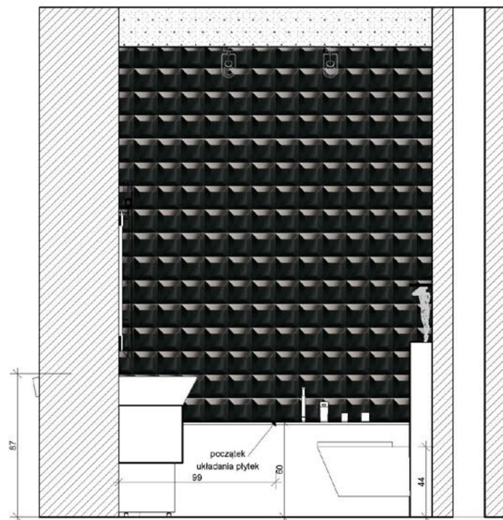
Łazienka 2 - przekrój C2
