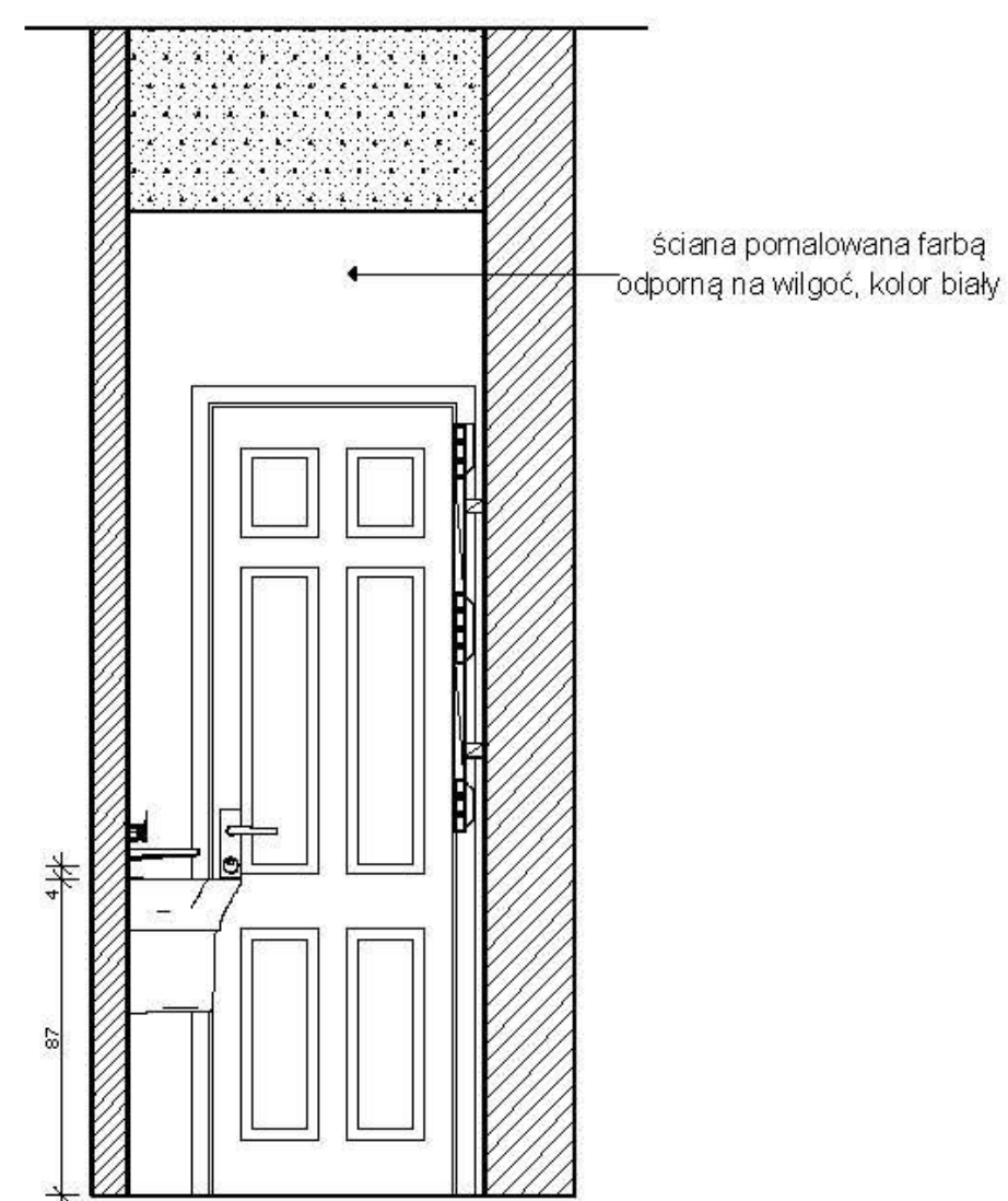
Łazienka 1 - przekrój B4
