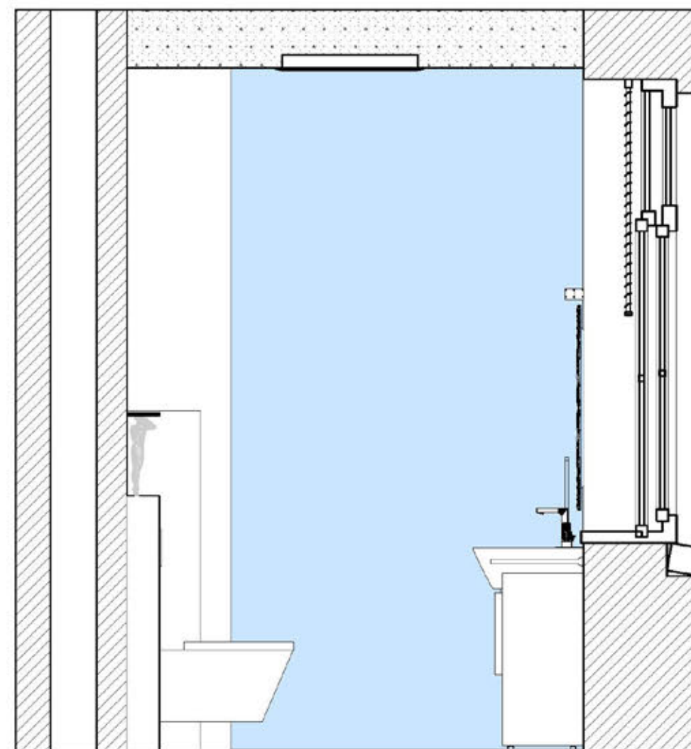
Łazienka 2 - przekrój C4
