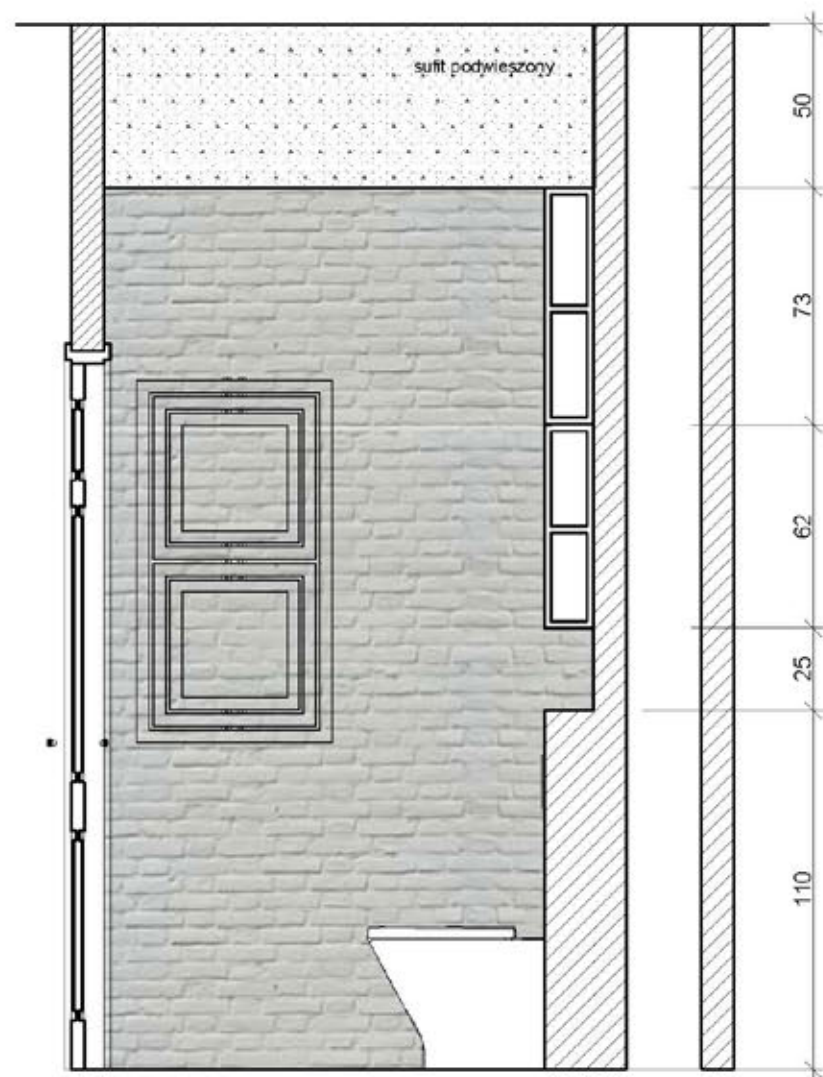
Łazienka 1 - przekrój B3
